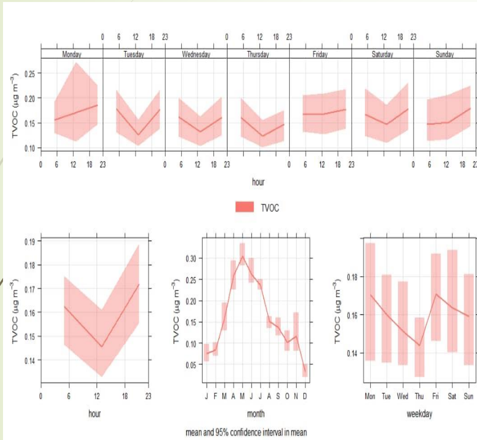
Figure 4. Profils temporels des COVT
