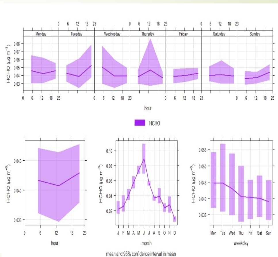
Figure 5. Profils temporels du HCOH
