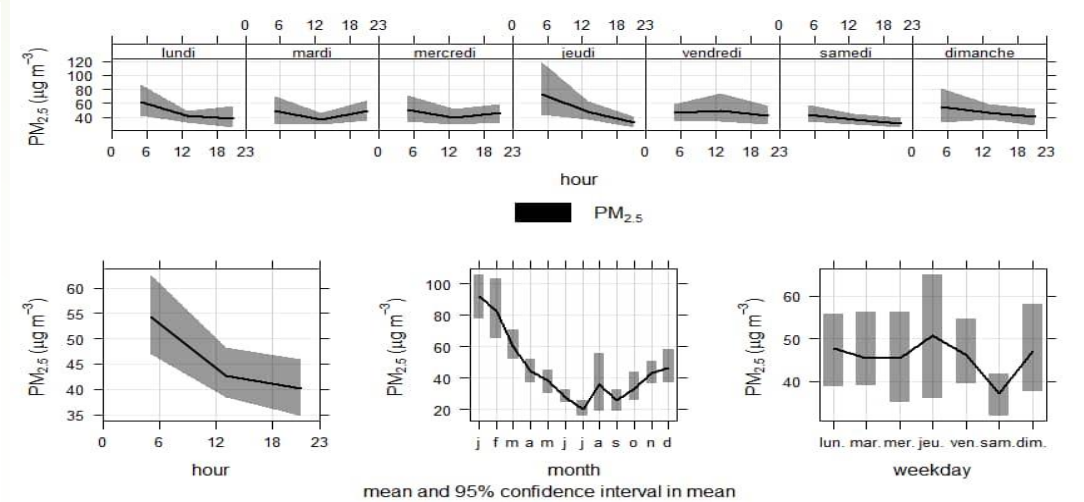
Figure 2. Profils temporels des PM_{2,5}
