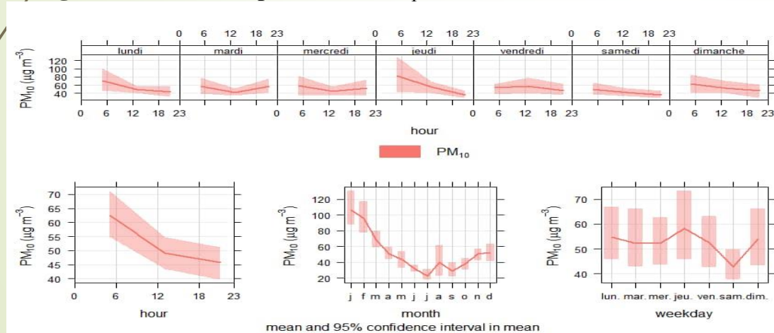
Figure 3. Profils temporels des PM_{10}
