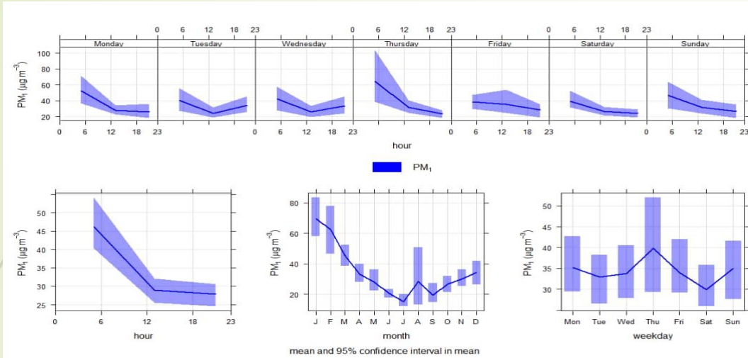
Figure 1. Profils temporels des PM_1
